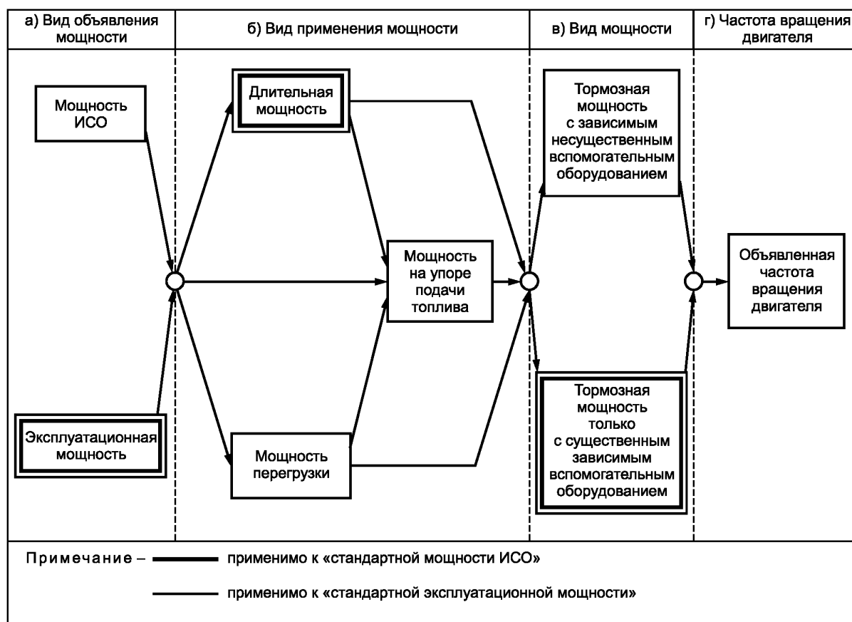
Рисунок 1 — Диаграмма, показывающая способы определения мощности
